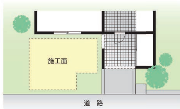
1台用 出幅違いタイプ
