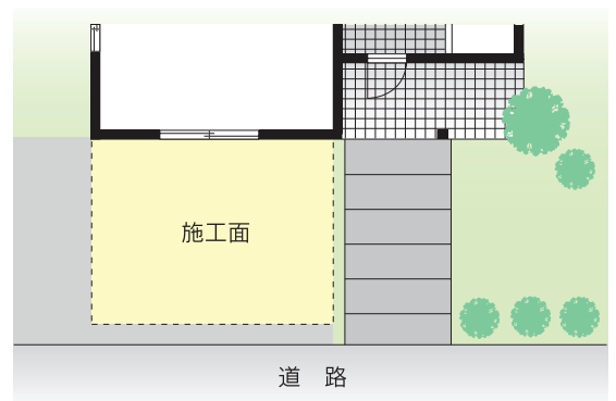
2台用 擁壁支持タイプ
