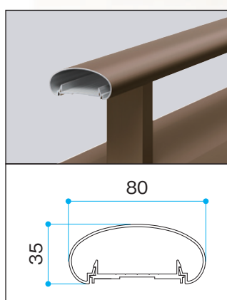
アルミ楕円手すり80
