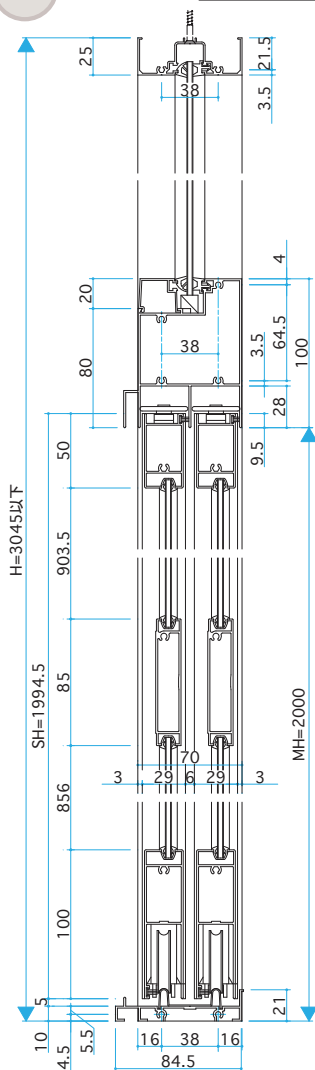
細框 ■MH=2000 A-A'断面
