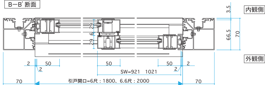
B-B' 断面
