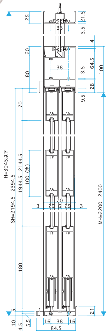
太框 ■MH=2200、2400 A-A'断面
