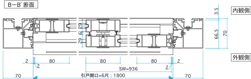
B-B' 断面
