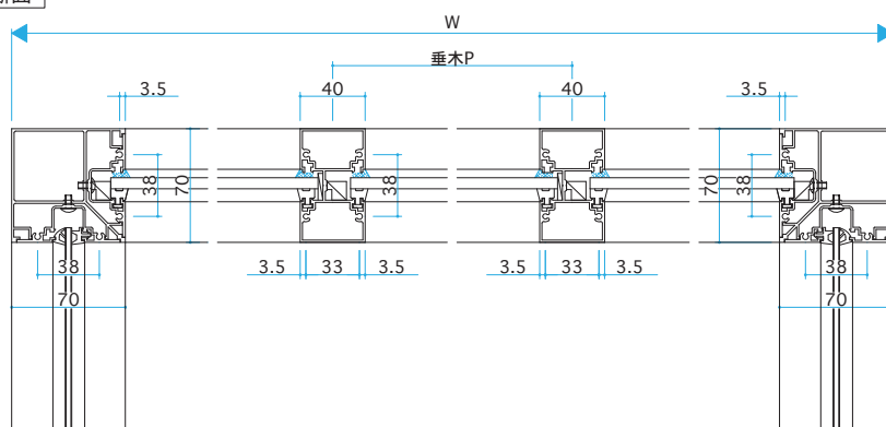
B-B' 断面
