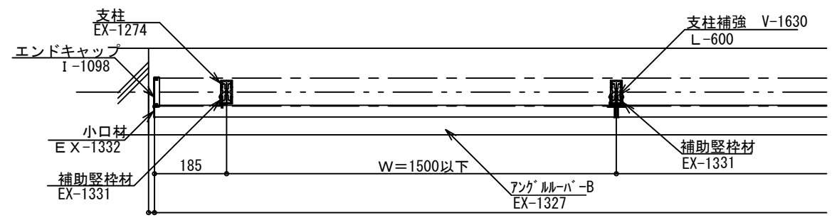
外開き 【姿図(内観図) 1/10】
