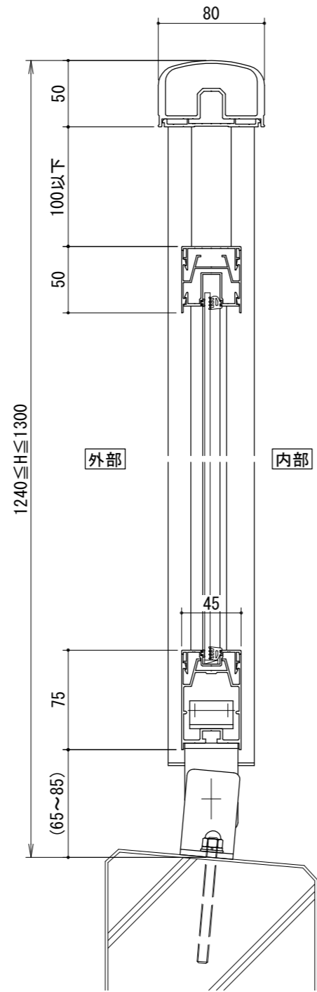
[二段手すりパネルタイプ]
