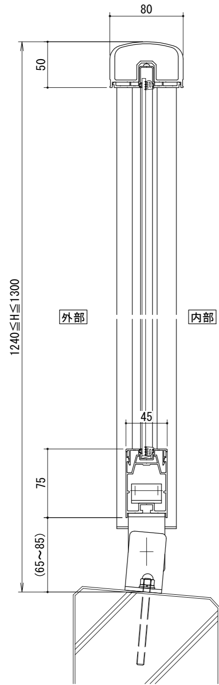
[一段手すりパネルタイプ]
