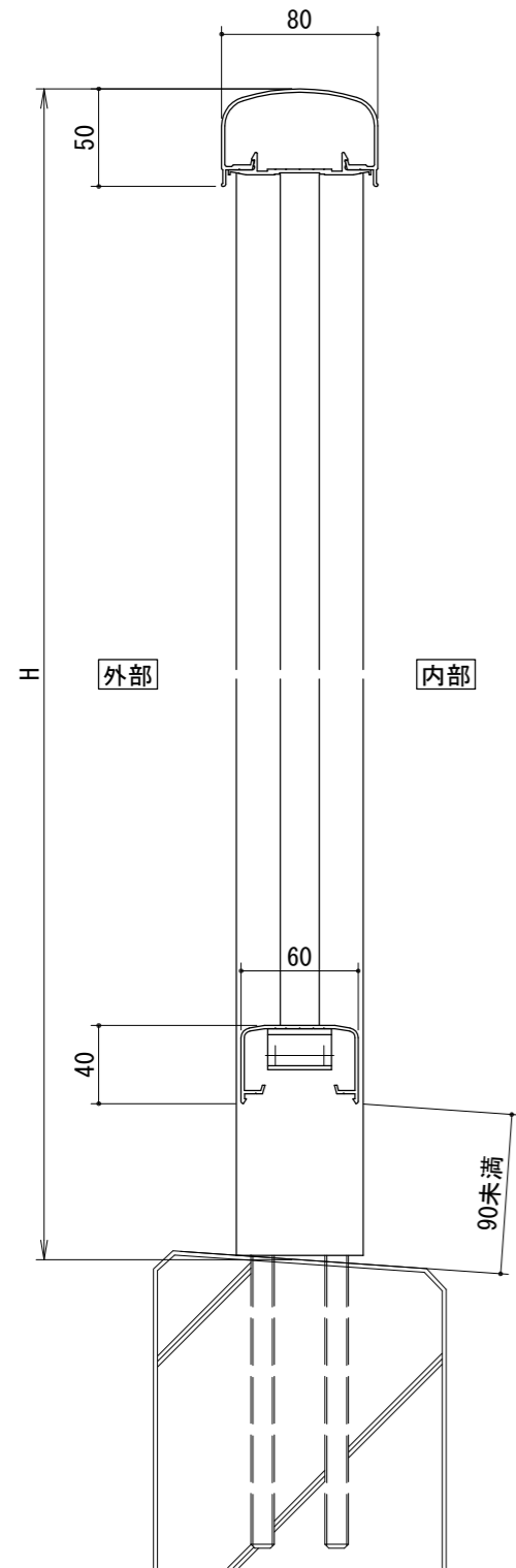
[一段手すりタテ格子タイプ]
