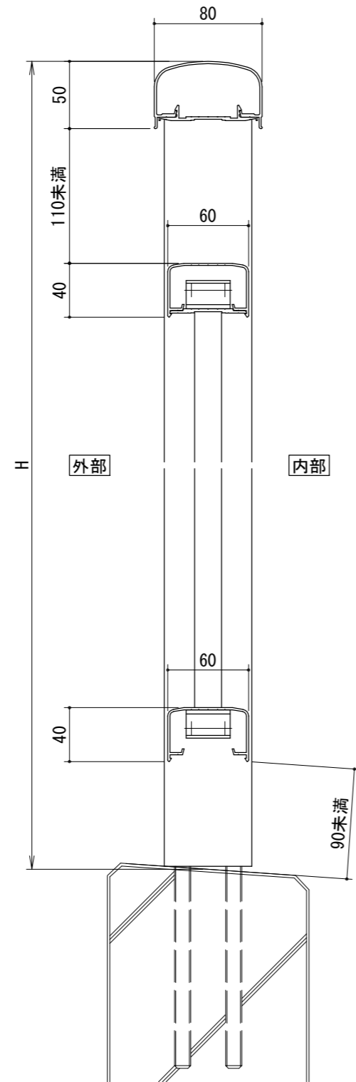
[二段手すりタテ格子タイプ]
