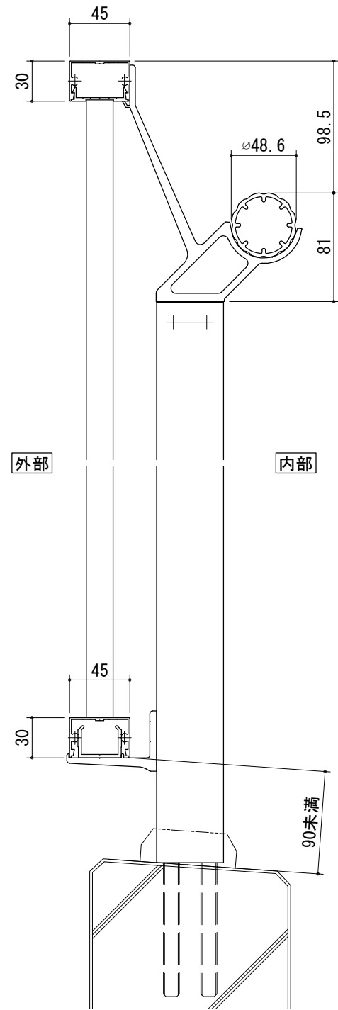
[タテ格子タイプ] 胴縁Lブラケット
