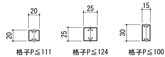
タテ格子バリエーション
