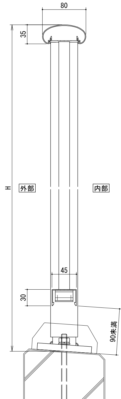
[一段手すりタテ格子タイプ]
