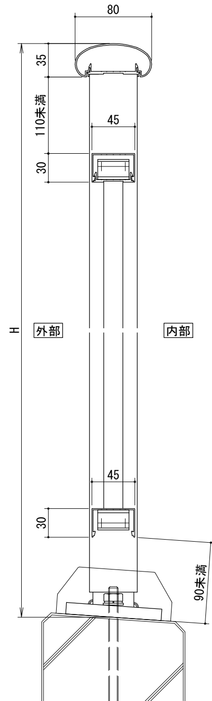
[二段手すりタテ格子タイプ]
