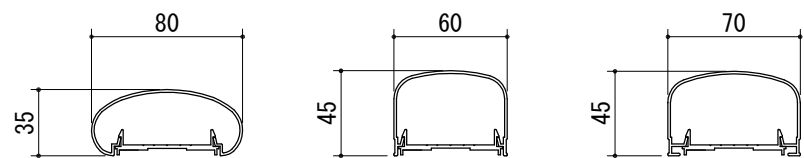
手すりバリエーション
