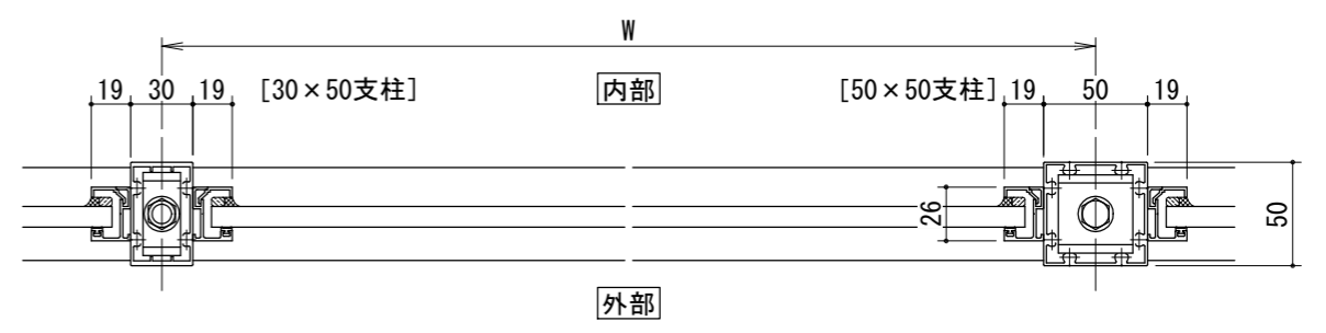
持ち出し納まり
