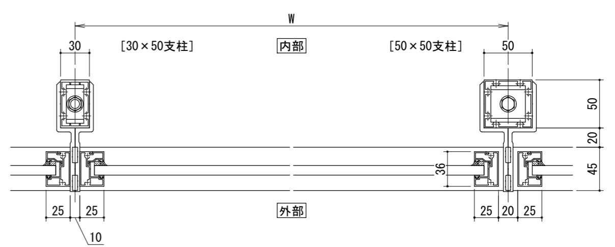
持ち出し納まり
