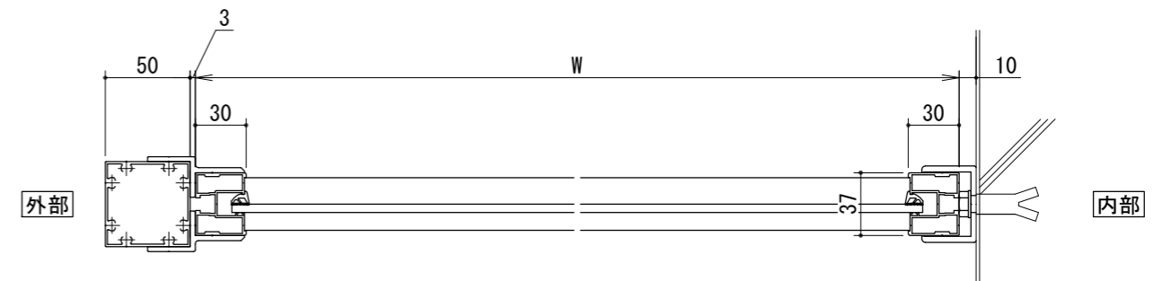
方立納まり
