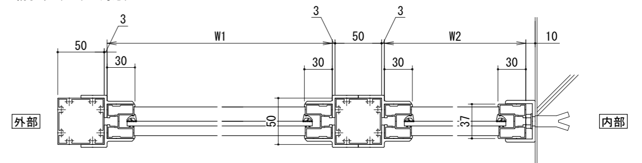
方立納まり (ワイド対応)
