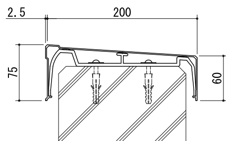
直線部
