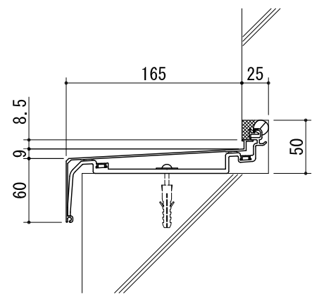
コーナー部
