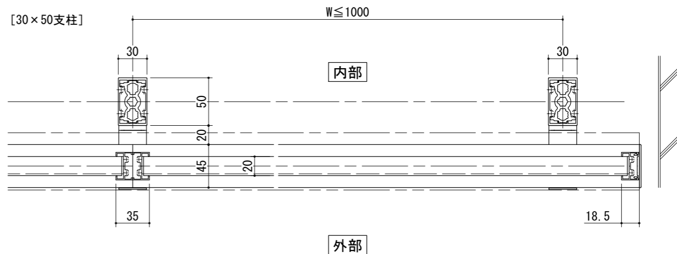
姿図(1:40)
