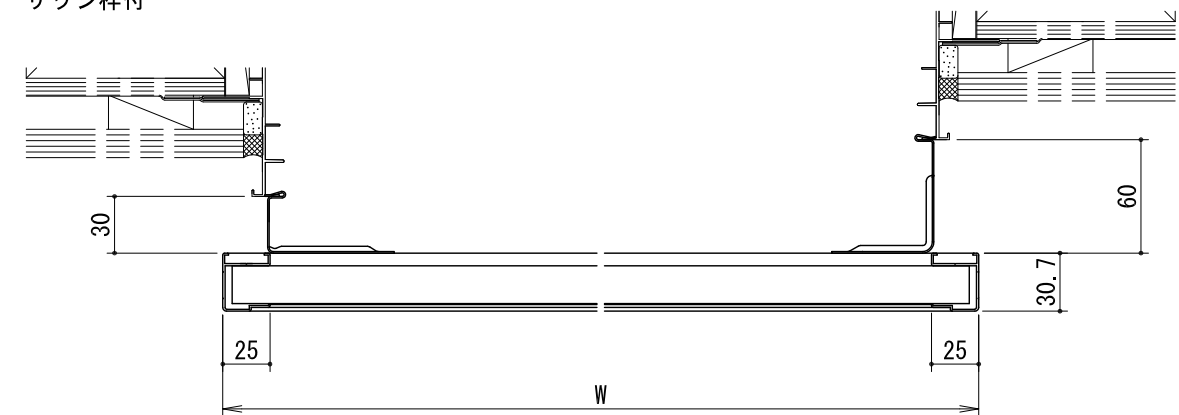
サッシ枠付
