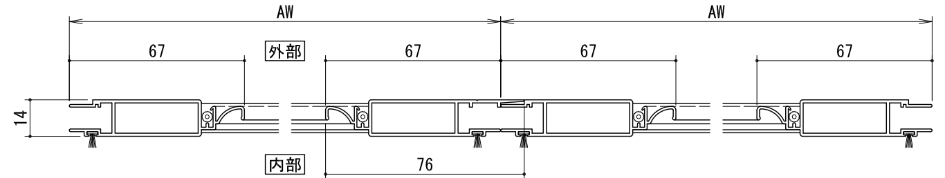
《4枚建の場合》
