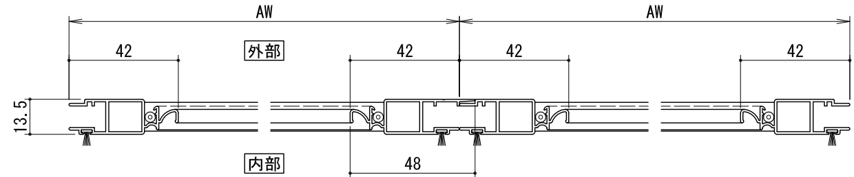
《4枚建の場合》
