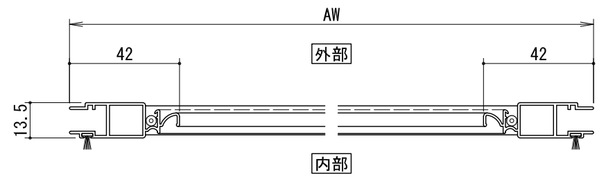
《2枚建の場合》
