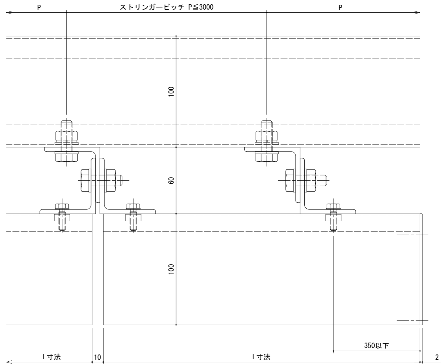
W断面
