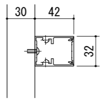
支柱間断面
