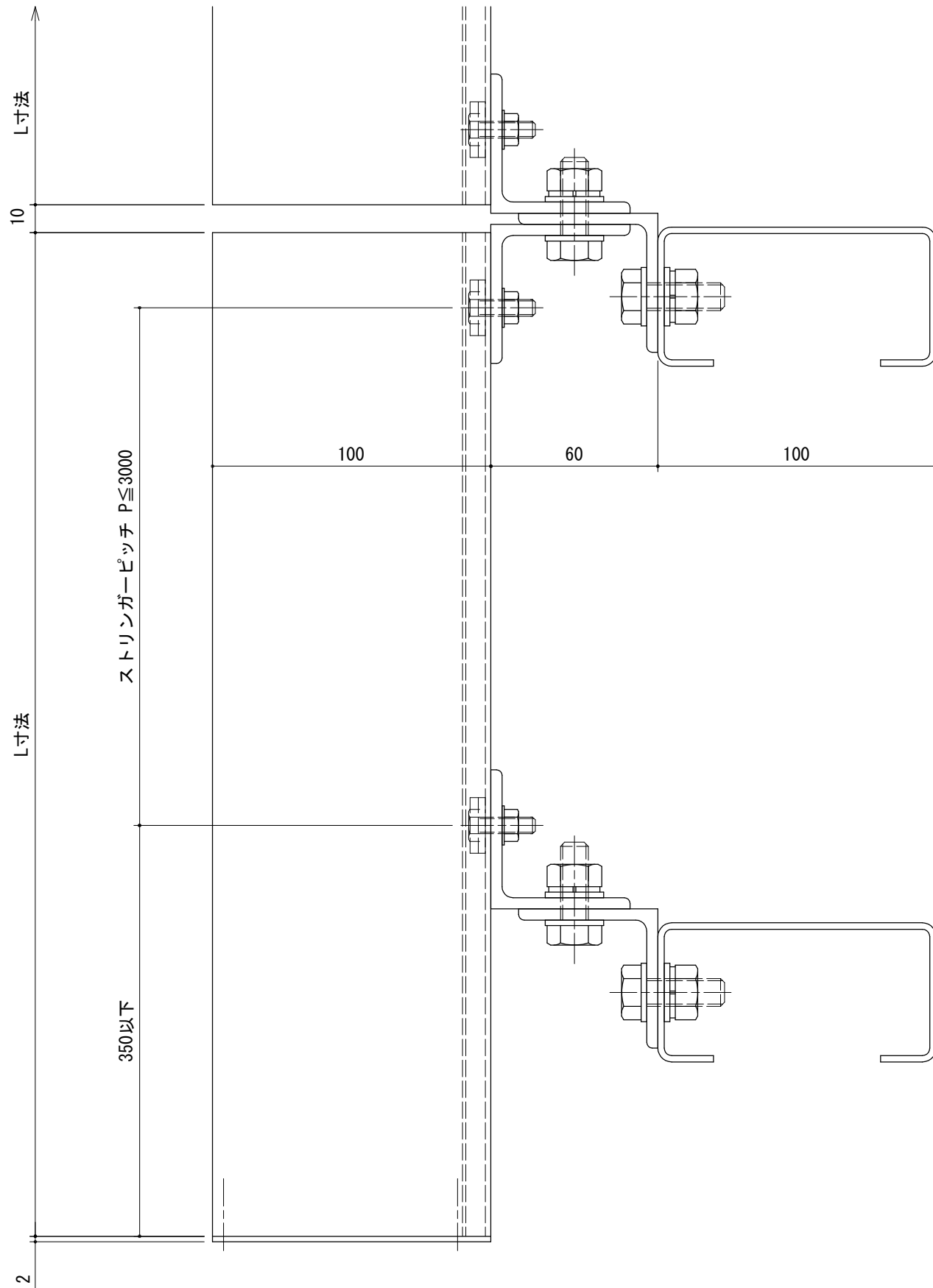
H断面
