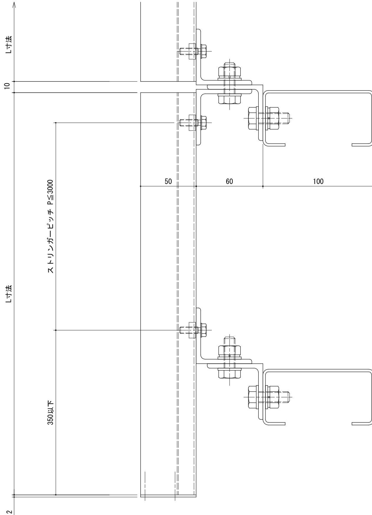
H断面
