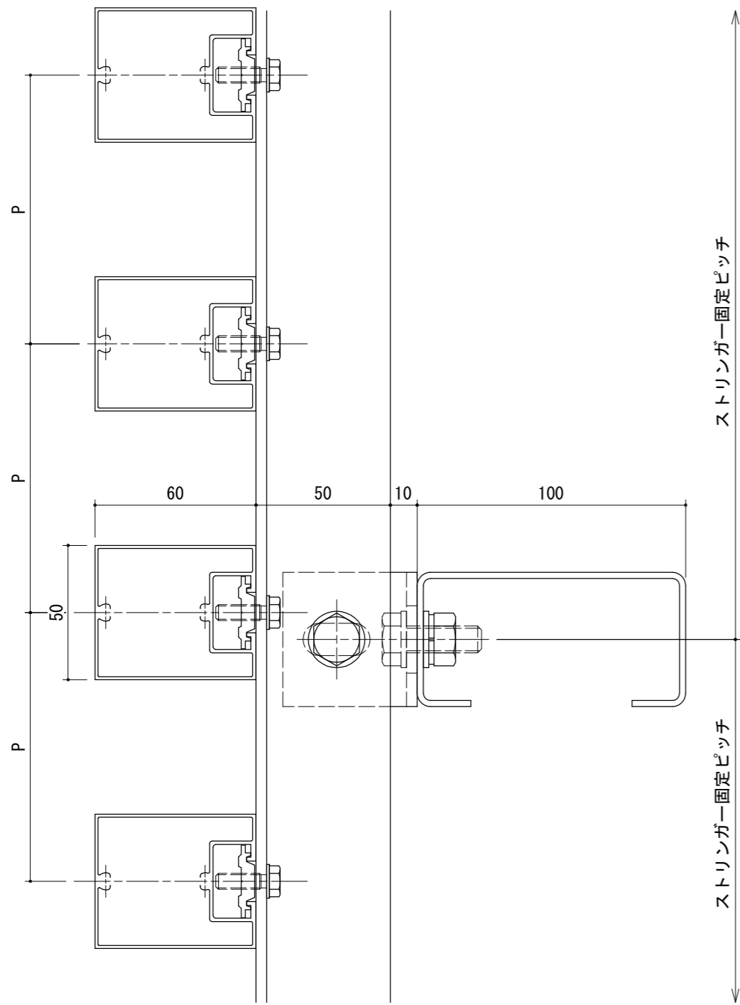
H断面
