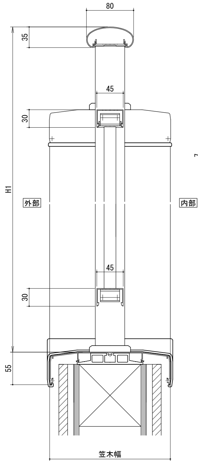
タテコーピング付
