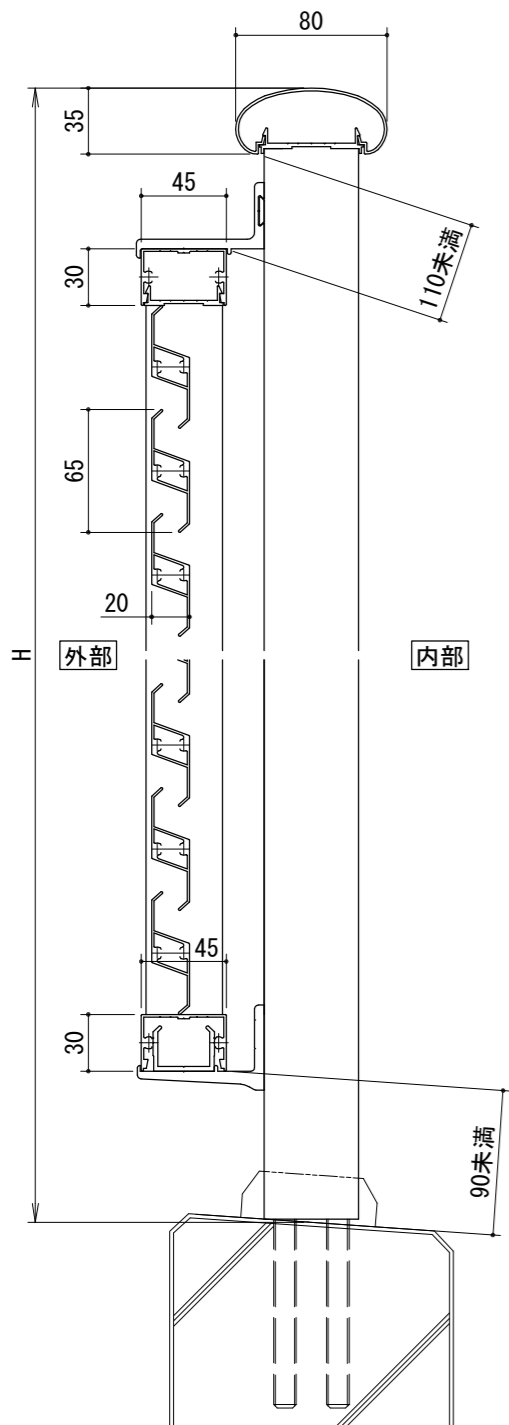
[ガラリタイプ] 胴縁Lブラケット
