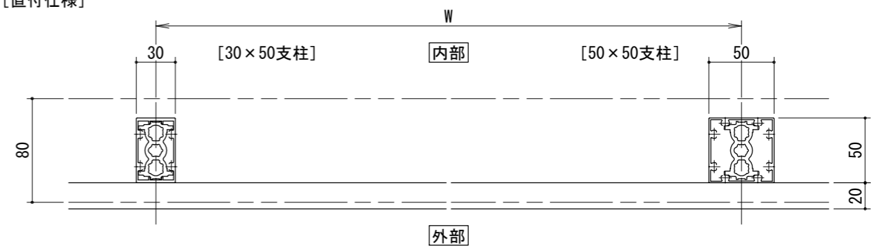
[直付仕様]
