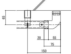
【手すりプラケット65エンド詳細】
