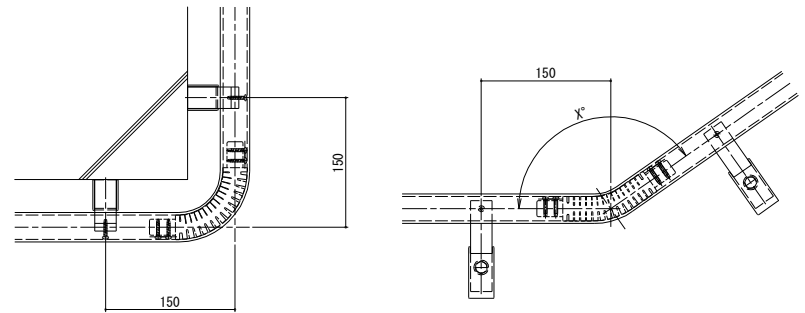
【手すりコーナー詳細】
