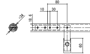
【レール材ジョイント詳細】
