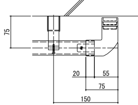
【手すりプラケット75エンド詳細】
