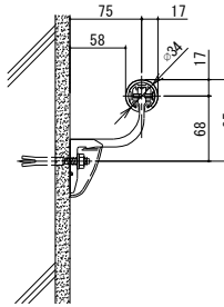
【手すりプラケット75】
