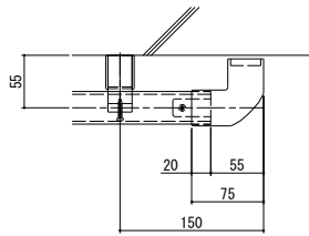
【手すりプラケット55エンド詳細】
