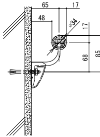
【手すりプラケット65】
