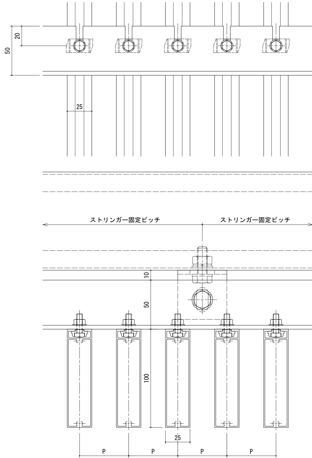
W断面
