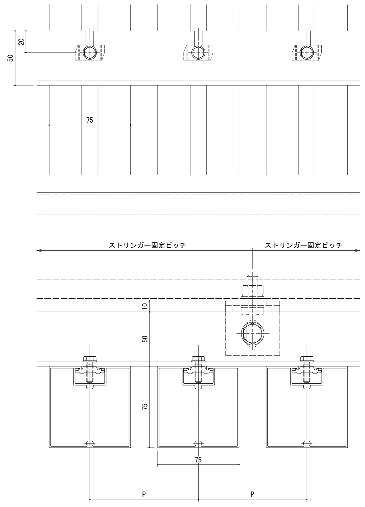
W断面
