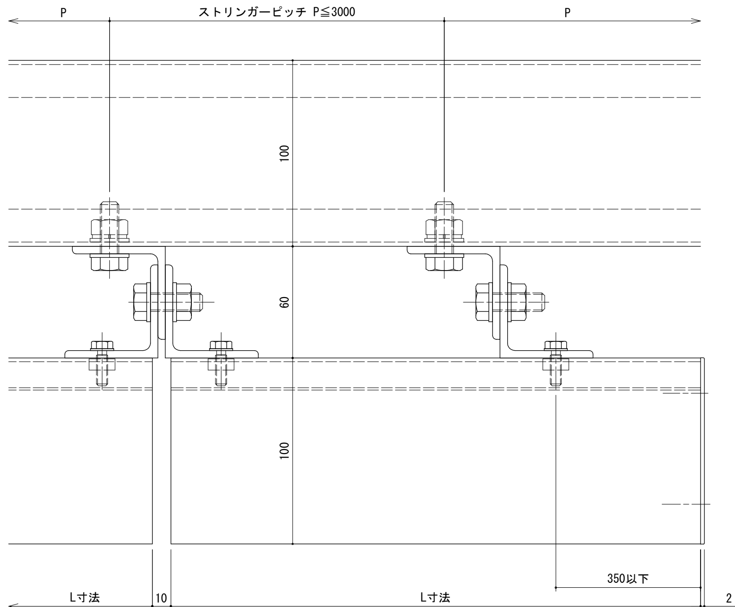
W断面
