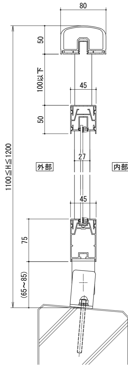
[二段手すりパネルタイプ]
