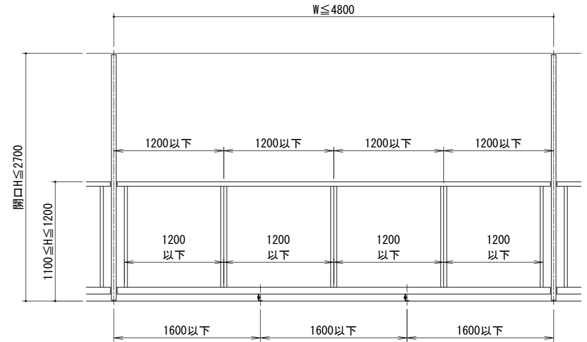
[一段手すりパネルタイプ]
