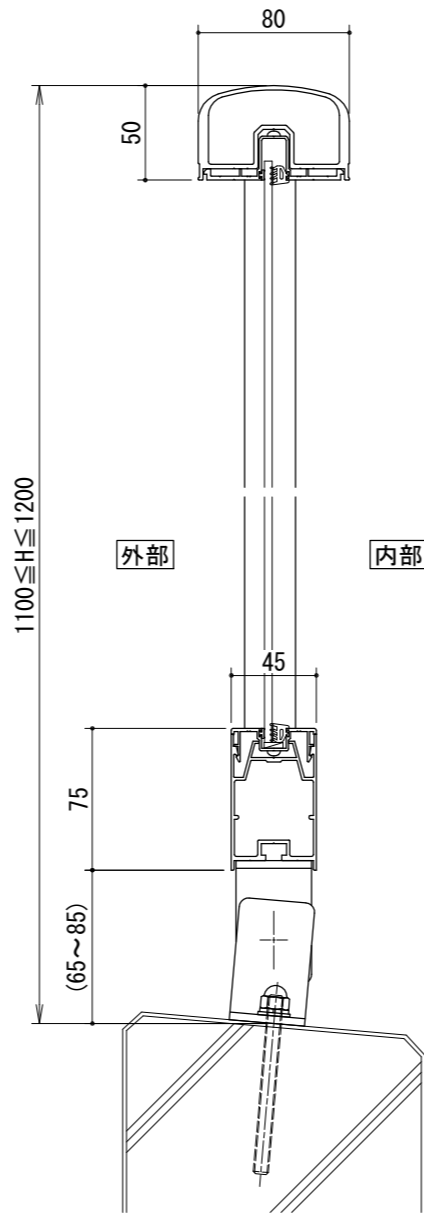
[一段手すりパネルタイプ]
