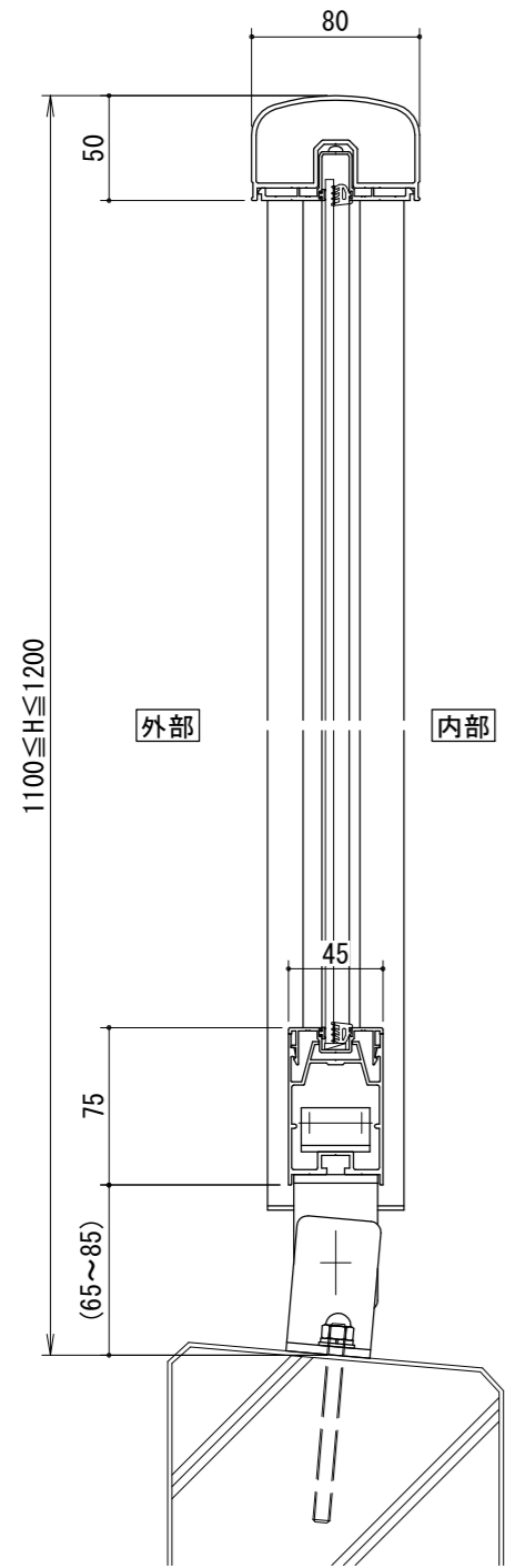
[一段手すりパネルタイプ]
