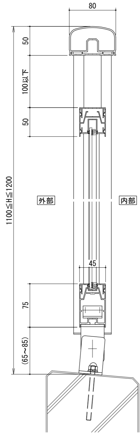
[二段手すりパネルタイプ]
