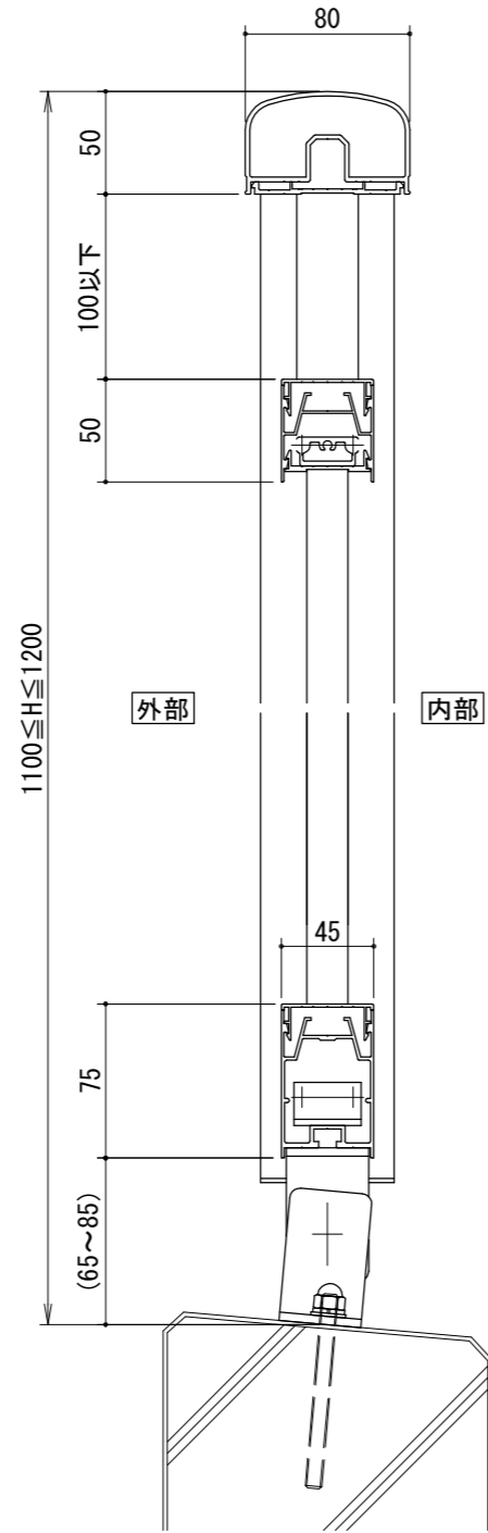
[二段手すりタテ格子タイプ]
