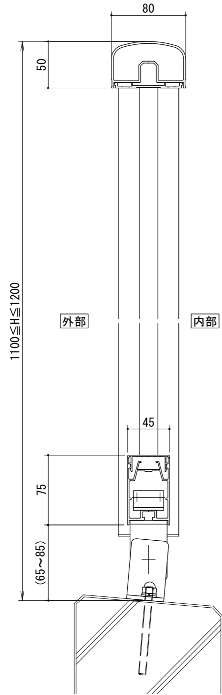
[一段手すりタテ格子タイプ]
