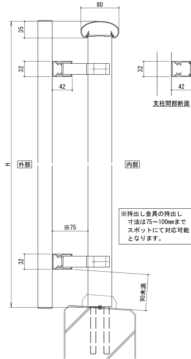
[タテ格子Aタイプ] ◎ステンレスブラケット仕様
