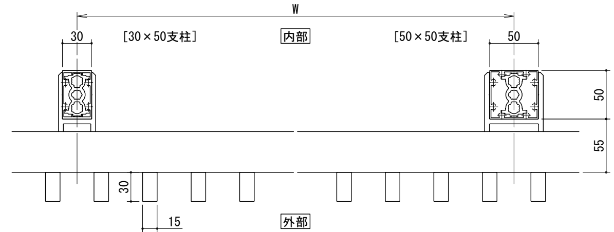
◎アルミブラケット仕様
