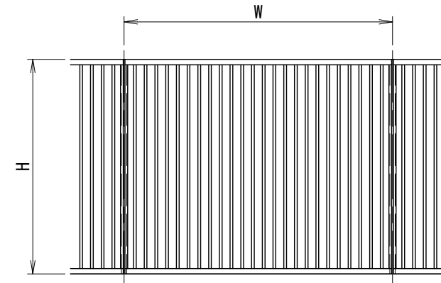
BL仕様 ※スラブ上納まり
