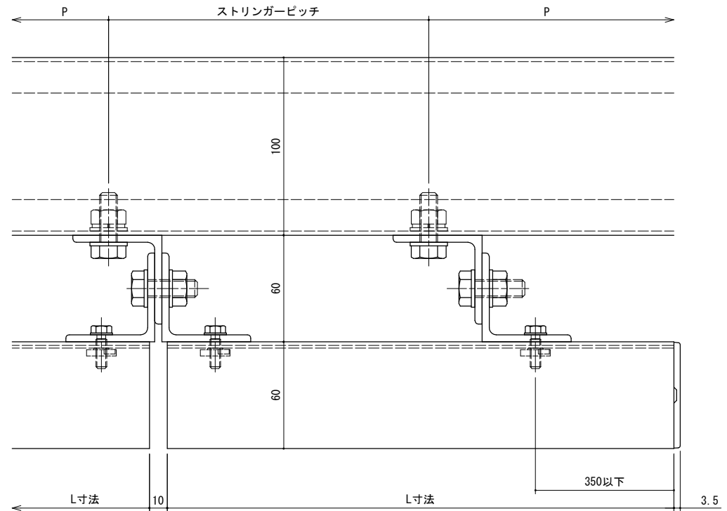
W断面
