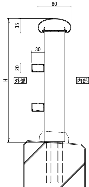
[横格子タイプ(持ち出し納まり)]
