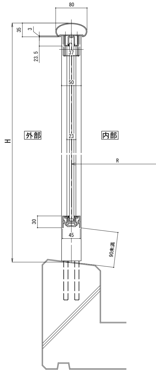
【一段手すりパネルタイプ】
