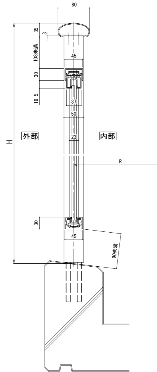
【二段手すりパネルタイプ】
