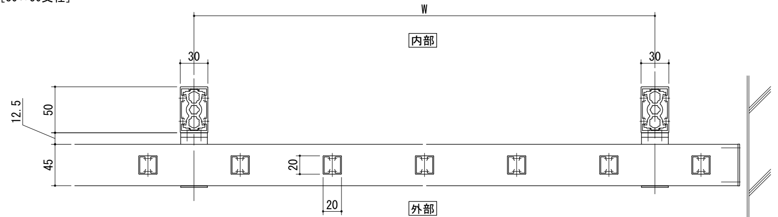
[30×50支柱]
