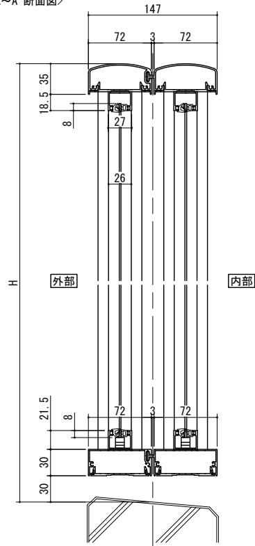
[1タイプ(パネルタイプ)] <A~A'断面図>
