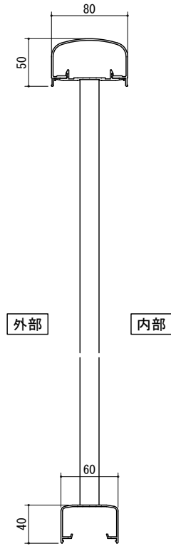
[一段手すりタテ格子タイプ] ※パネルタイプ対応不可
