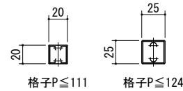
タテ格子バリエーション
