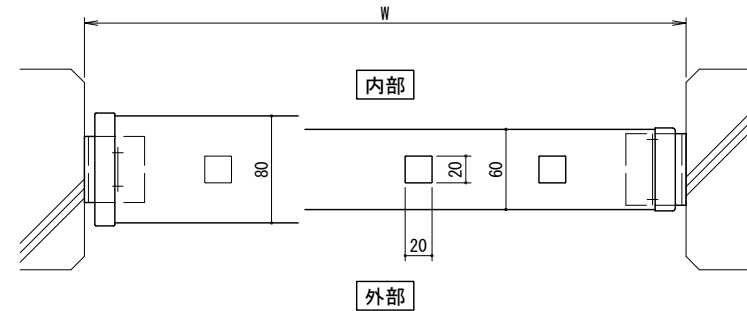
タテ格子バリエーション
