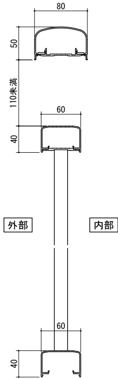
[二段手すりタテ格子タイプ] ※パネルタイプ対応不可
