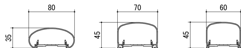
手すりバリエーション
