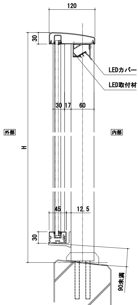
【縦断面】 基準図
