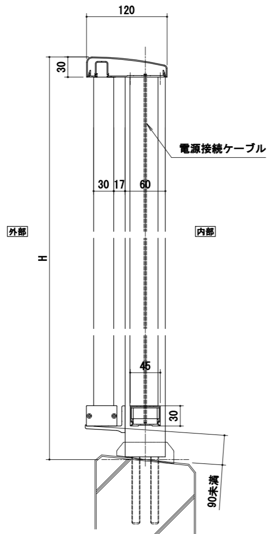
【縦断面】 給電部
