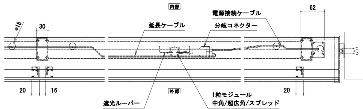
【平面図(胴縁部)】
