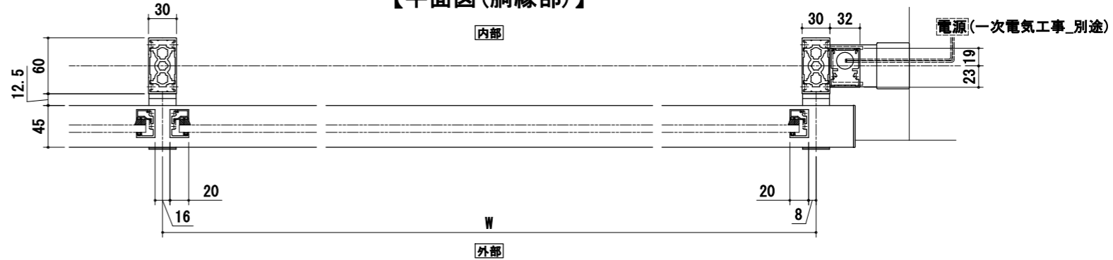
【平面図(胴縁部)】
