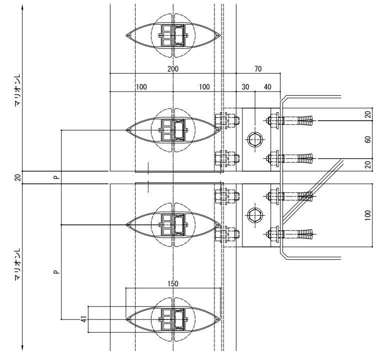
B部詳細図
