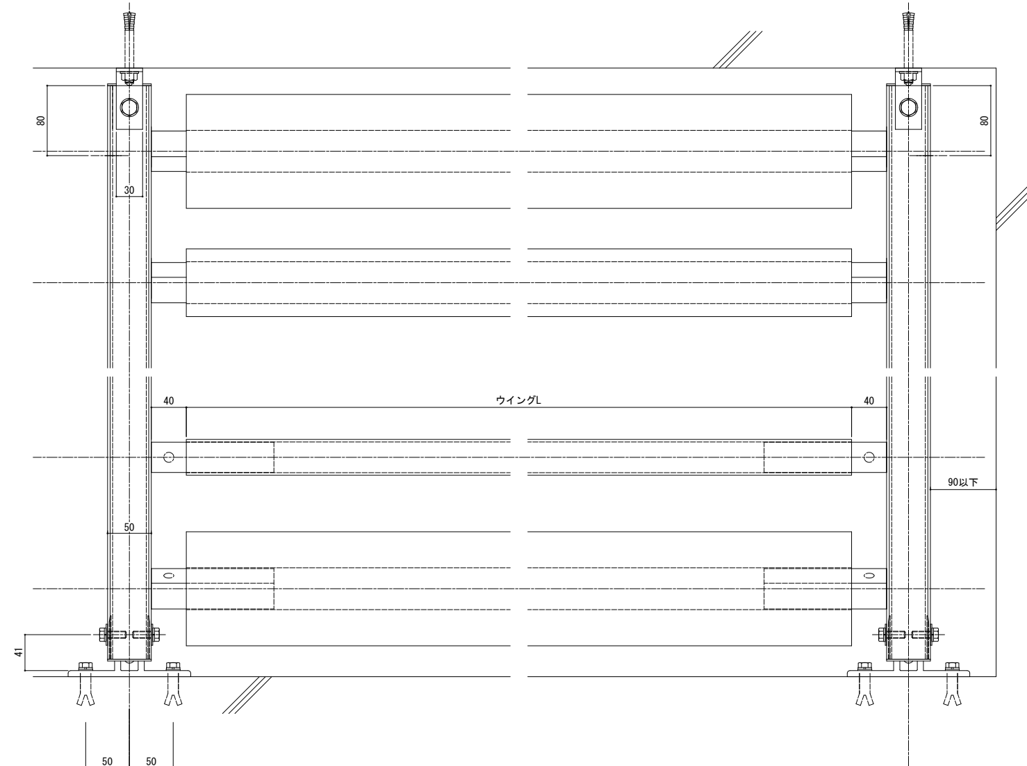
【外観姿図】
