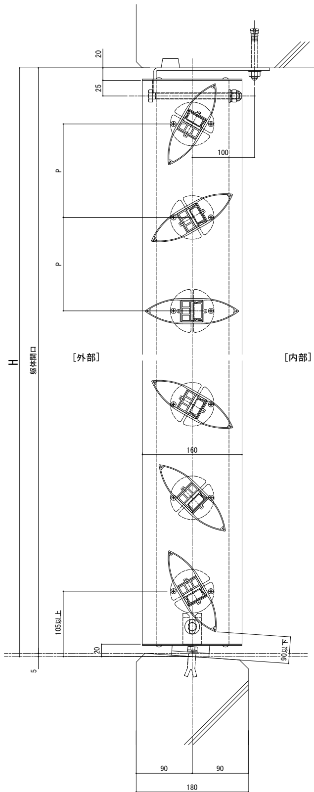
【縦断面図】
