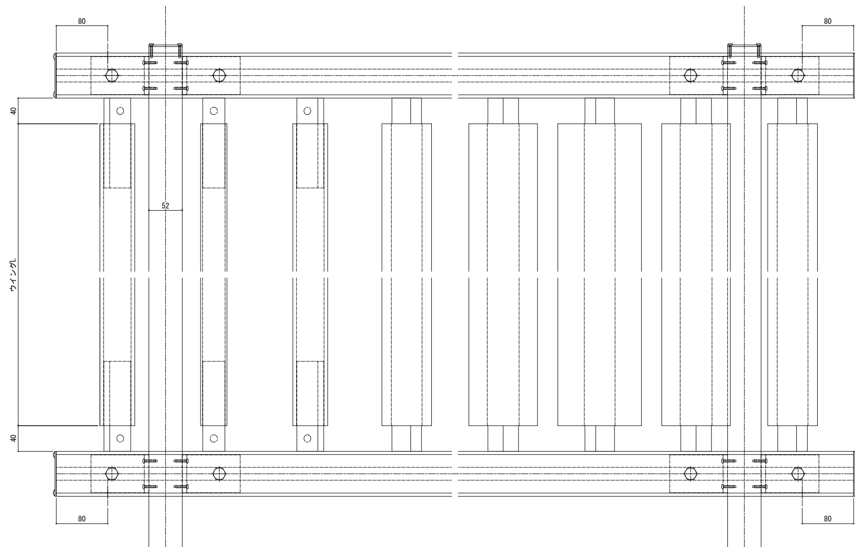
【外観姿図】
