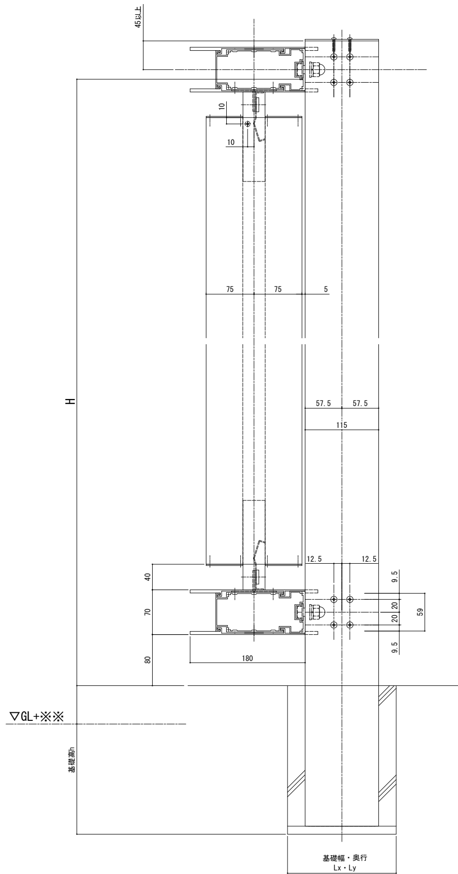
【縦断面図】
