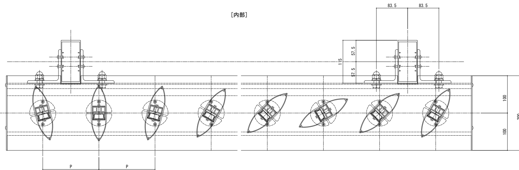
【横断面図】
