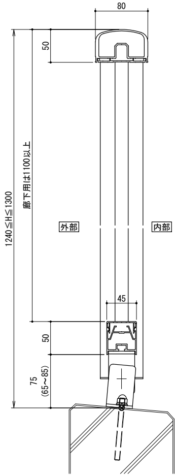
[一段手すりタテ格子タイプ]
