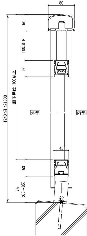
[二段手すりタテ格子タイプ]
