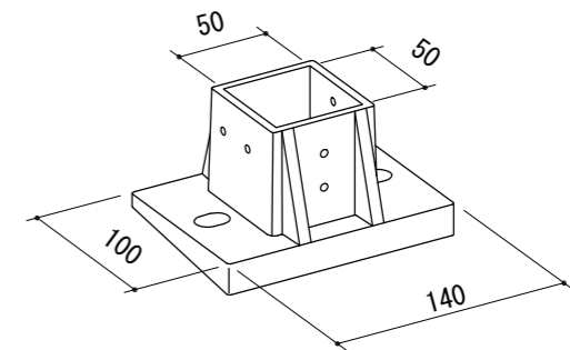
【支柱ベース】
