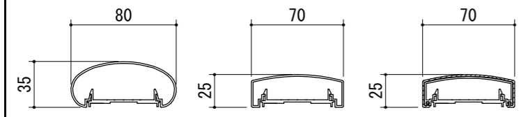
手すりバリエーション
