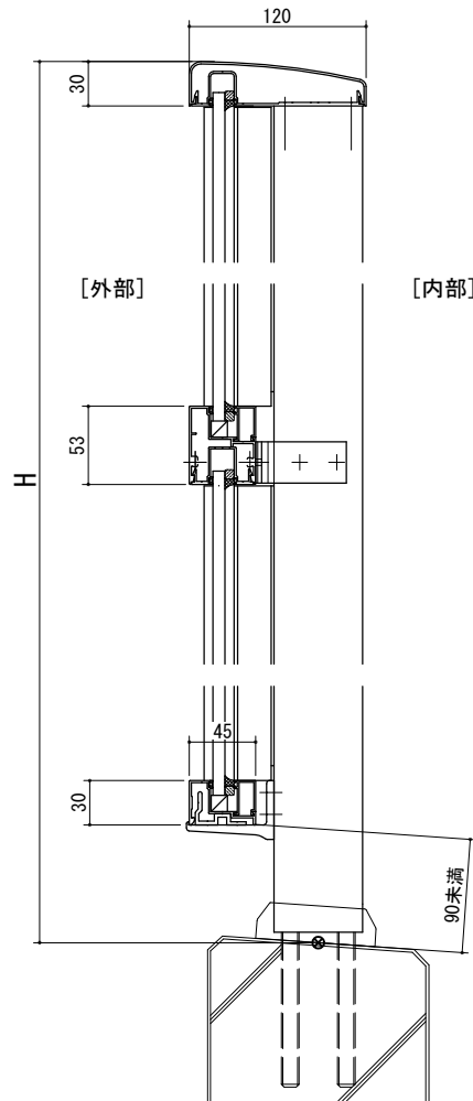
[上下ガラス縦枠Aタイプ] 中間
