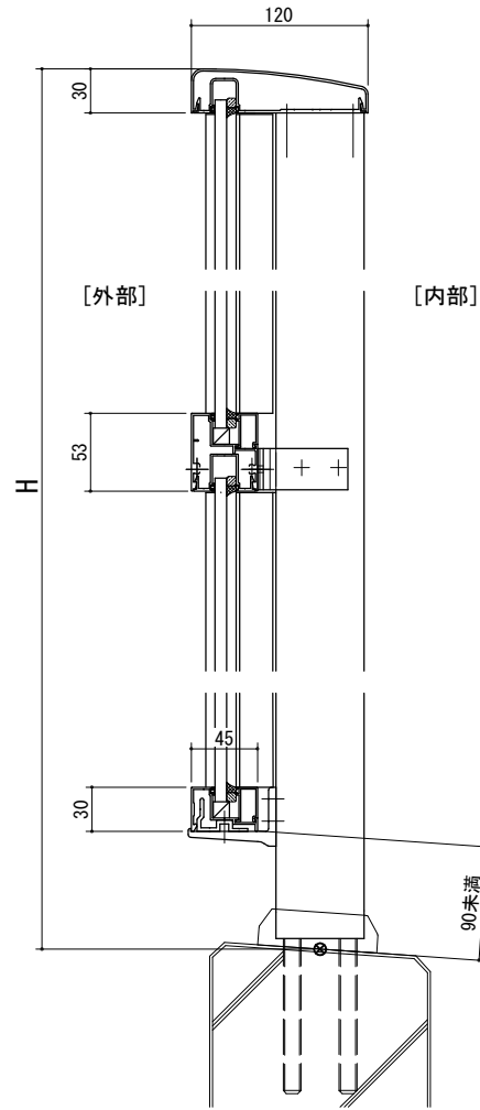
[上下ガラス縦枠Aタイプ] 端部
