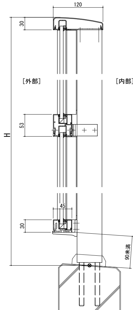
[上下ガラス縦枠Bタイプ] 中間
