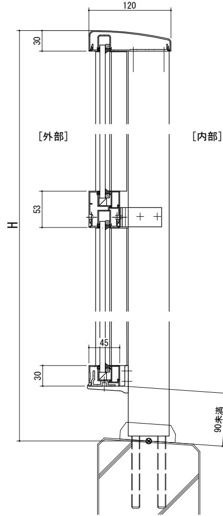
[上下ガラス縦枠Bタイプ] 端部
