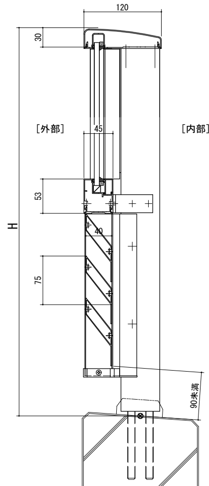
【上ガラス（竖枠B）下ルーバータイプ】 中間
