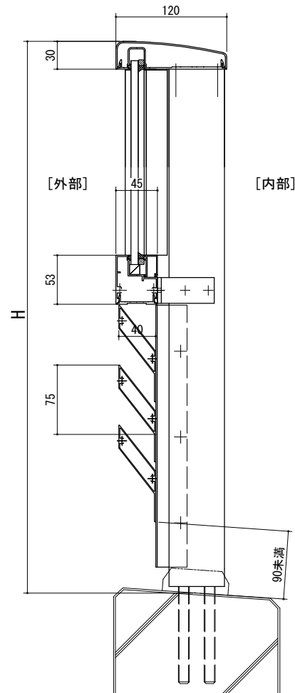
【上ガラス（竖枠B）下ルーバータイプ】 端部
